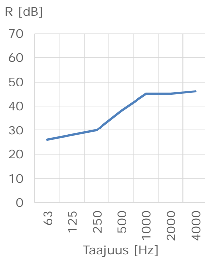
Kuva 3.8. Erään 80-luvulla rakennetun pientalon makuuhuoneen julkisivun ilmaääneneristävyys. Rakenteena on tiilijulkisivu, jossa on yksi 2 m 2 kokoinen ikkuna. Mittaus on tehty ISO 140-5 mukaan (Työterveyslaitos).
